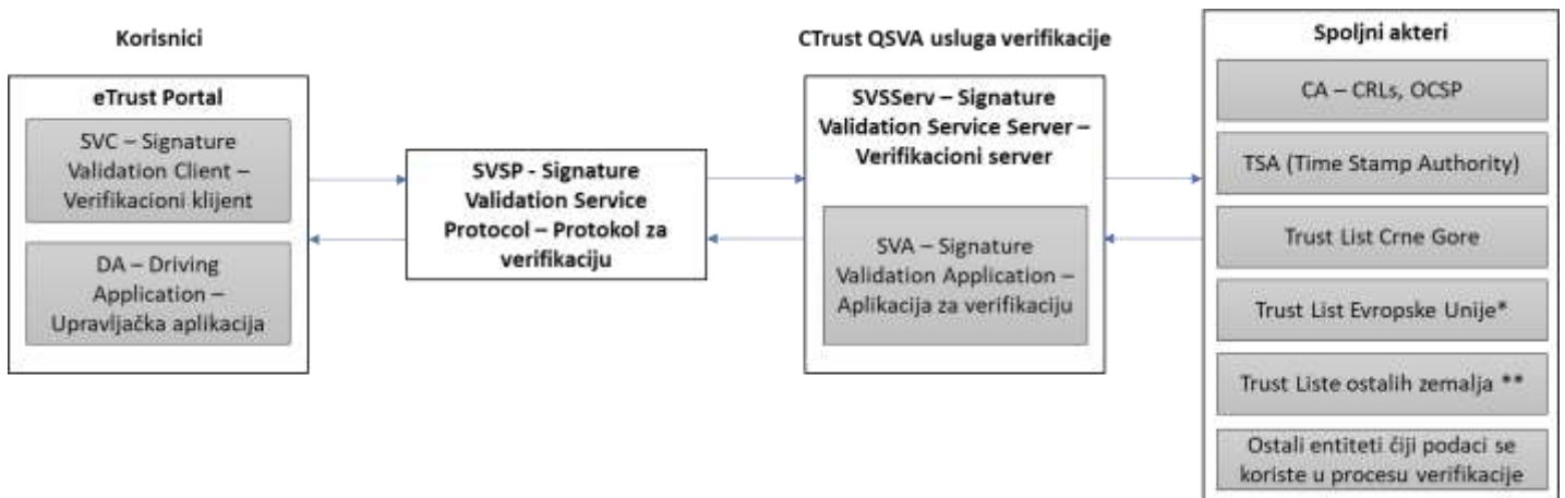
Slika 1. – Arhitektura usluge za verifikaciju
