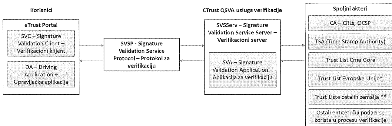
Slika 1. – Arhitektura usluge za verifikaciju
