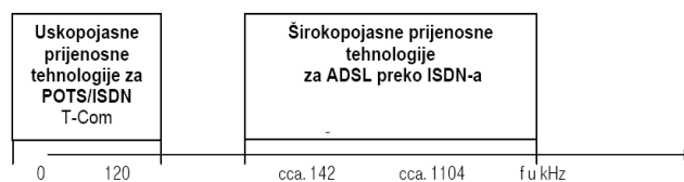
Slika 1. Frekvencijski obim za uskopojasne i širokopolasne prenosne tehnologije
