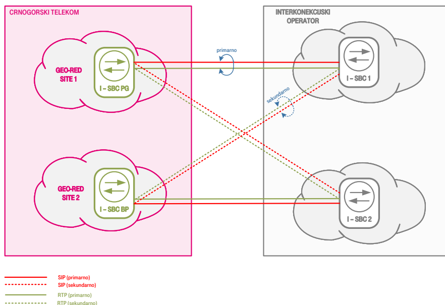
Slika 2 – Arhitektura povezivanja mreže CT sa interkonekcionim partnerom sa dva I-SBC-a (usmjeravanje saobraćaja po hunt principu)
